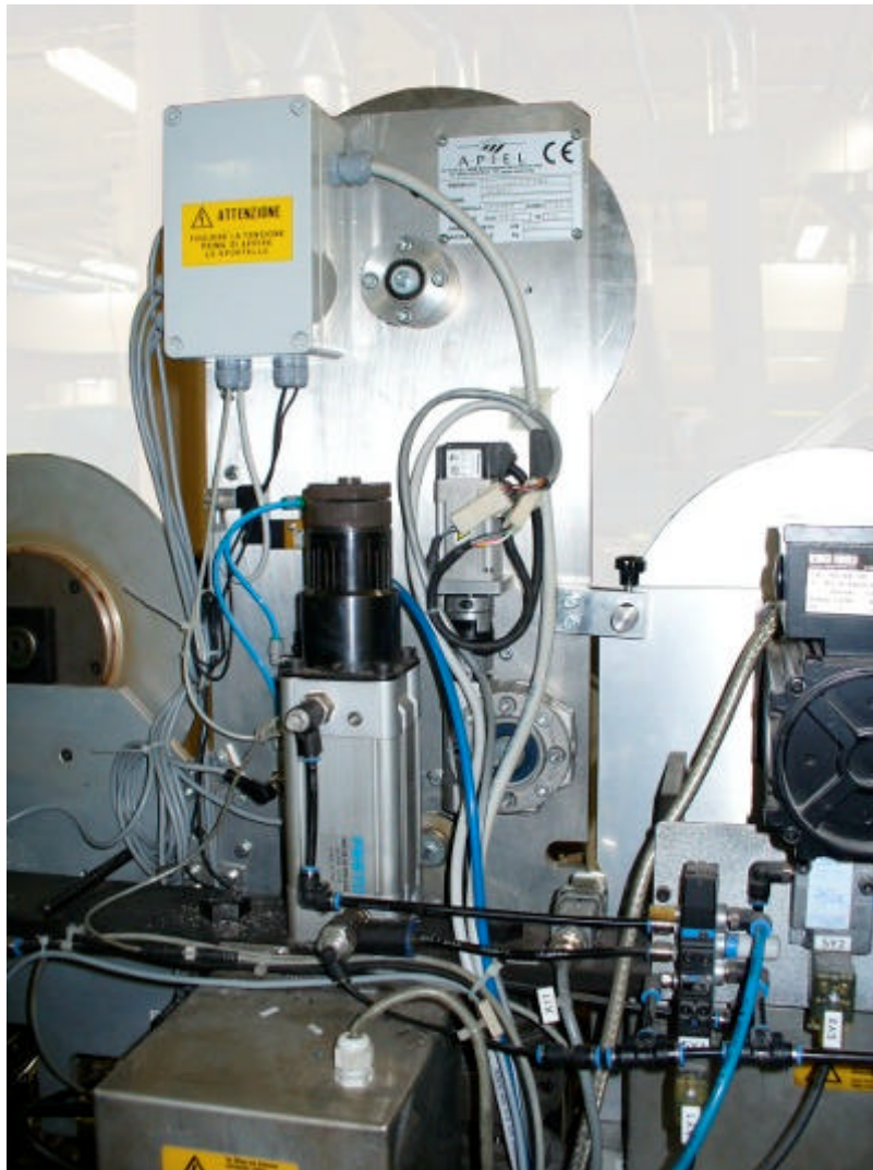
Vista posteriore del gruppo di recupero scratch off
