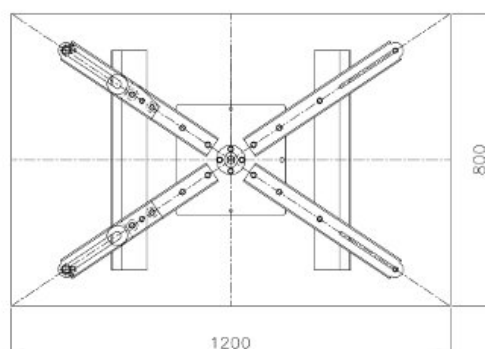
Elemento di presa con ventose
