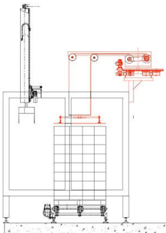
Mettifalda a rotaia esempio posizionamento su pallettizzatore cartesiano
